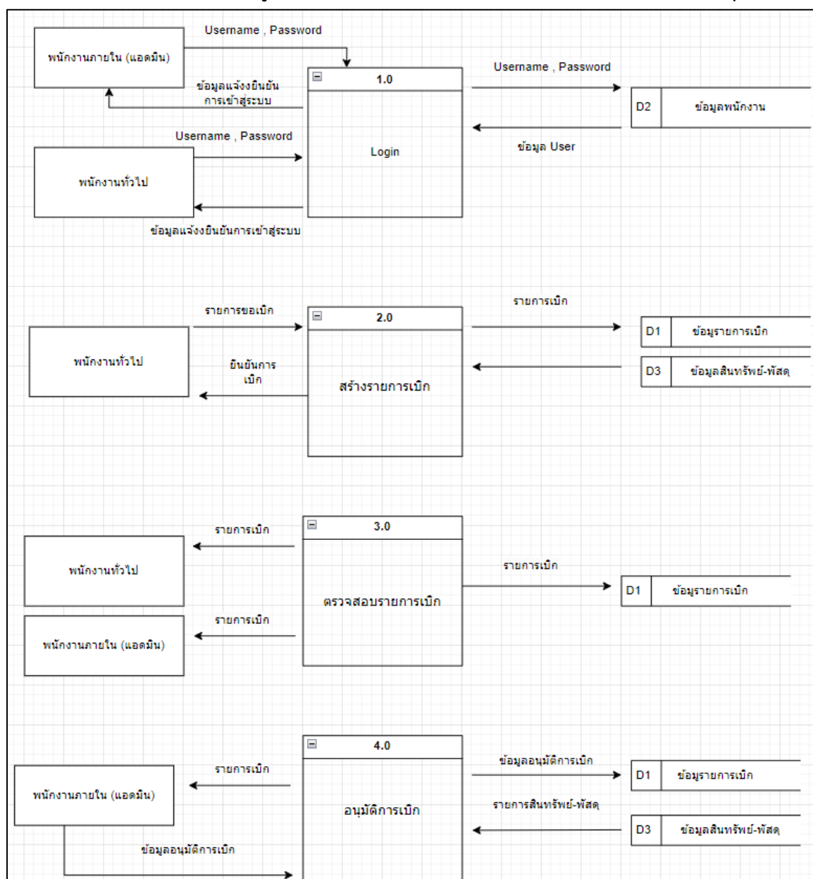
รูป ค.4 ( Data flow diagram ) ของระบบการเบิกสินทรัพย์-พัสดุ
