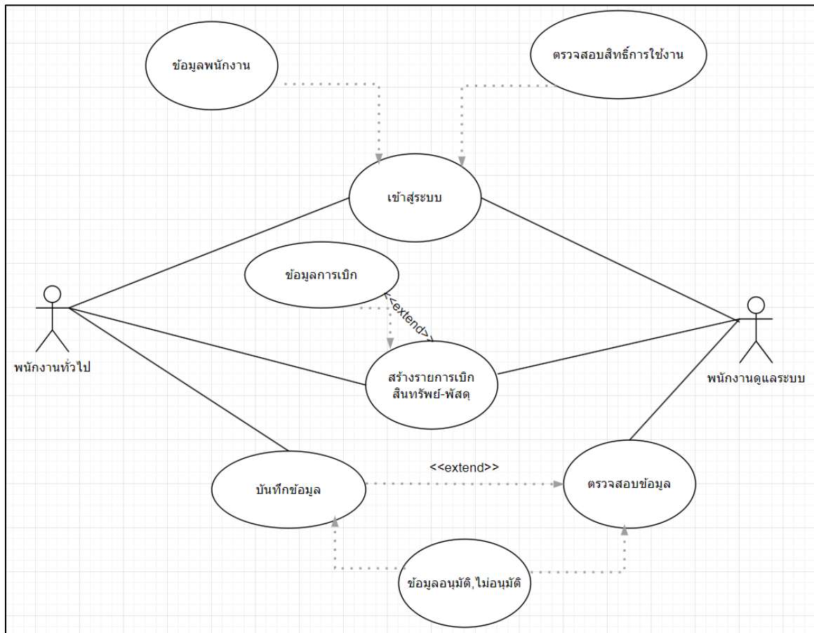
รูปที่ ค.1 แผนภาพแสดงการทำงานของผู้ใช้ระบบ Use case Diagram
