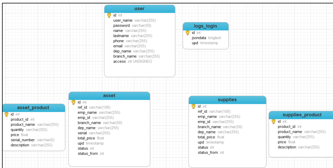
รูปที่ ค.6 ER Diagram ระบบการเบิกสินทรัพย์ – พัสดุ
