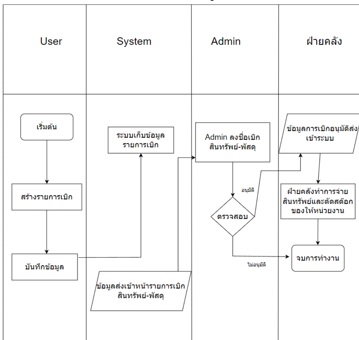
รูปที่ ค.2 Flowchart กระบวนการสร้างรายการเบิก
